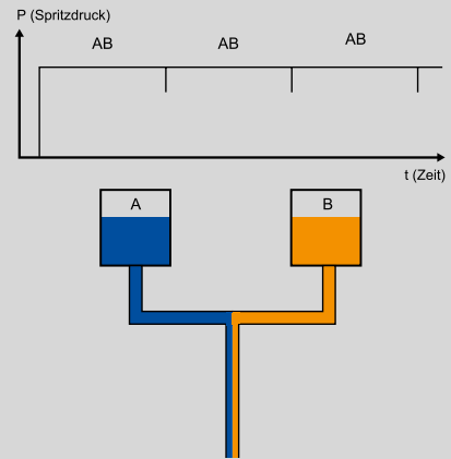
WIWA DUOMIX Kontinuierliche Dosierung
