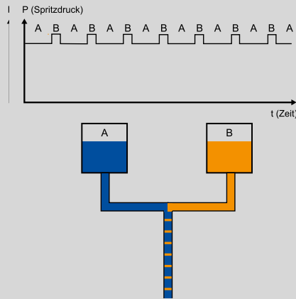
WIWA FLEXIMIX II Kurze Taktzeiten
