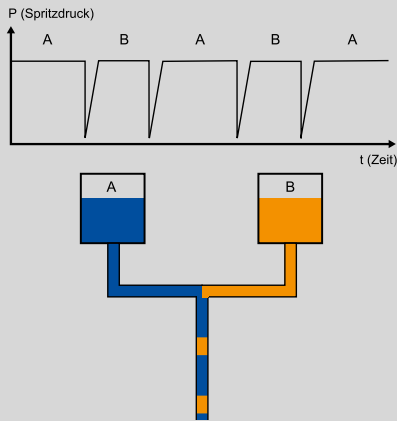
Variable Wettbewerbs-2K-Anlage Lange Taktzeiten
